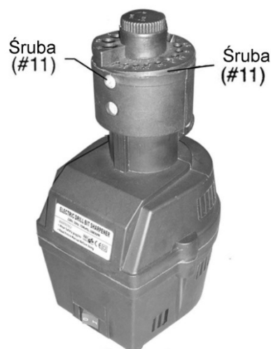
Rysunek 4: Odkręcanie śrub
