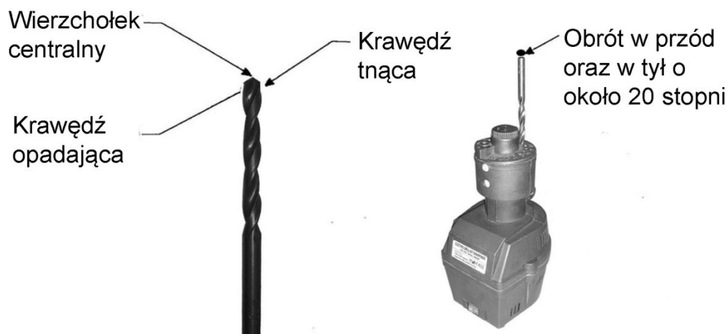
Rysunek 1: Elementy wiertła
